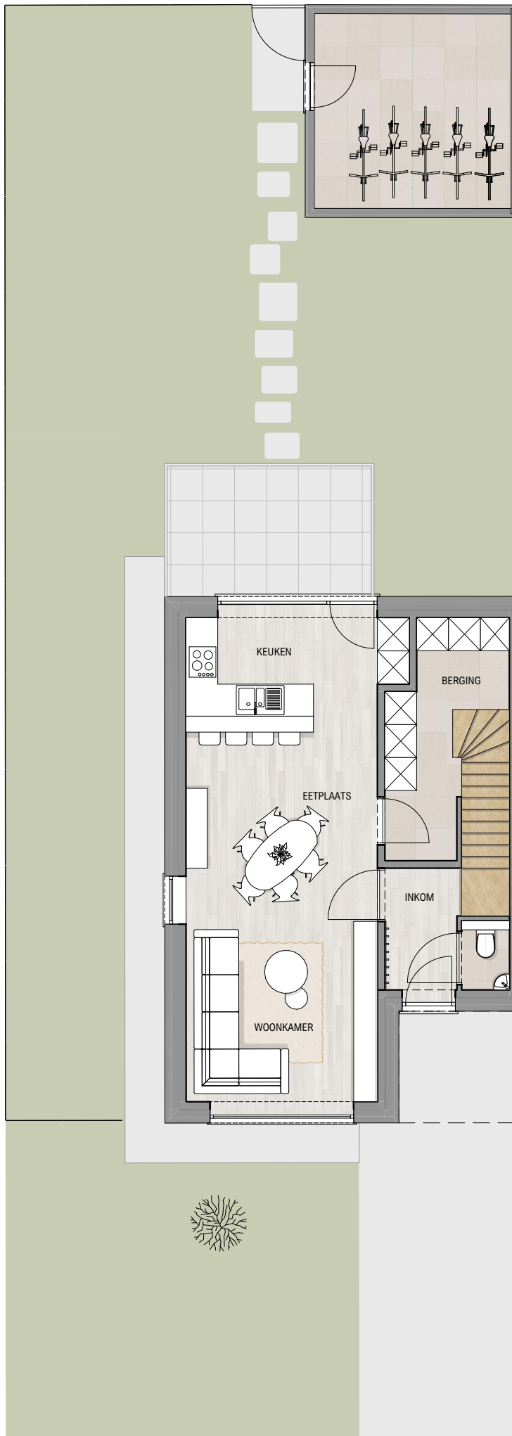
GELIJKVLOERS
